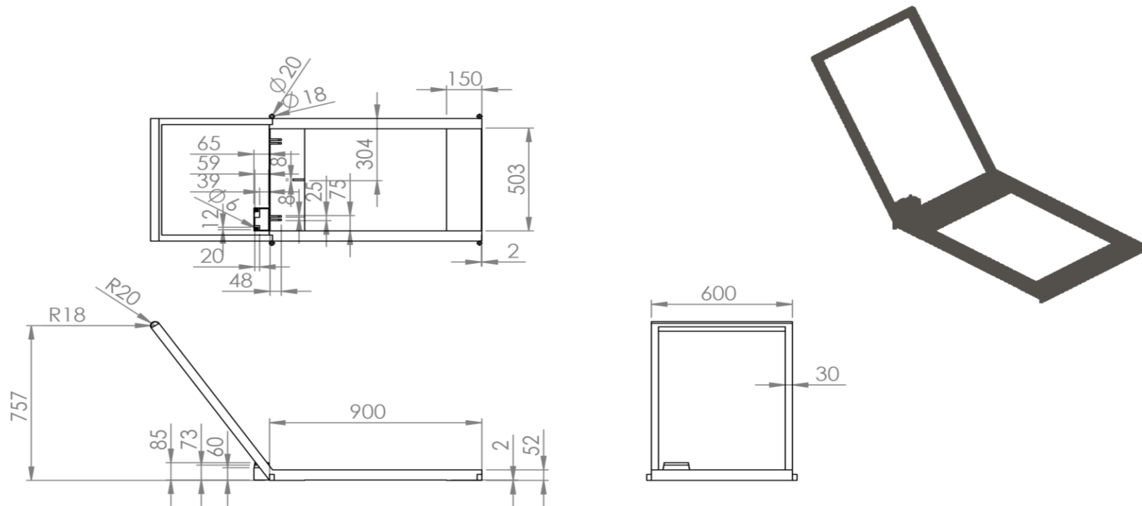
Lampiran 1 Gambar Kerja Rangka Utama
