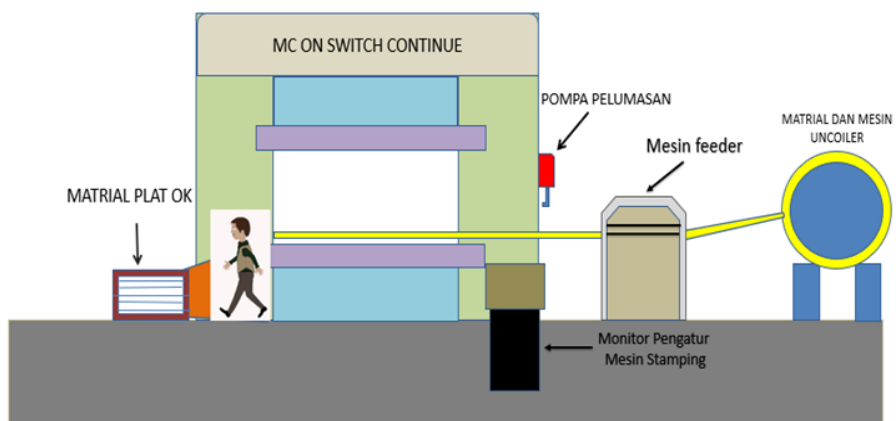
VISUALISASI SESUDAH PEMBUATAN POMPA PELUMASAN OTOMATIS
