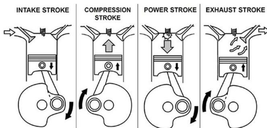
Gambar 2.2 prinsip kerja motor bensin (Nugrahadi, 2023)
