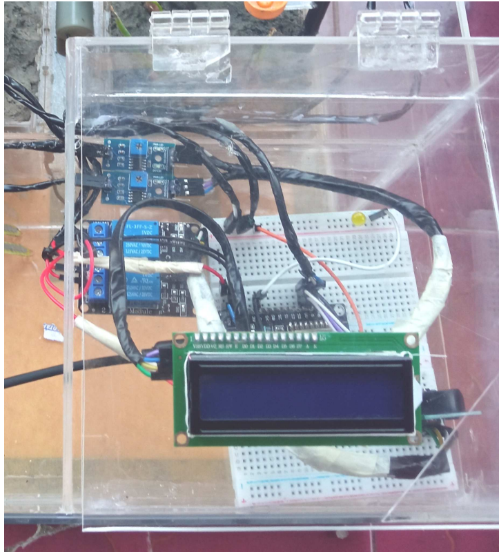
Gambar 5. 3 Rangkaian Sistem Pengairan dan Pencahayaan Otomatis
