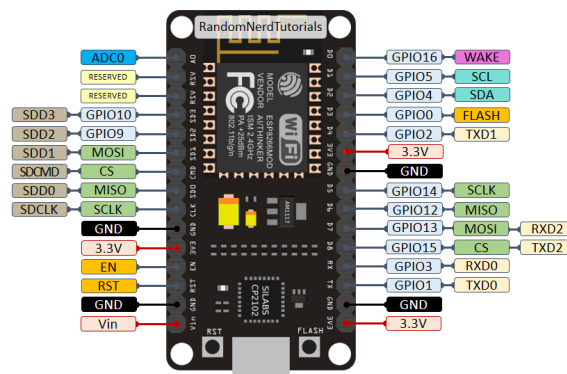
Gambar 2. 1 Konfigurasi Pin NodeMCU ESP8266 V3
